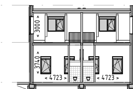
Langsdoorsnede
