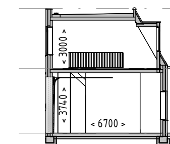
Dwarsdoorsnede
