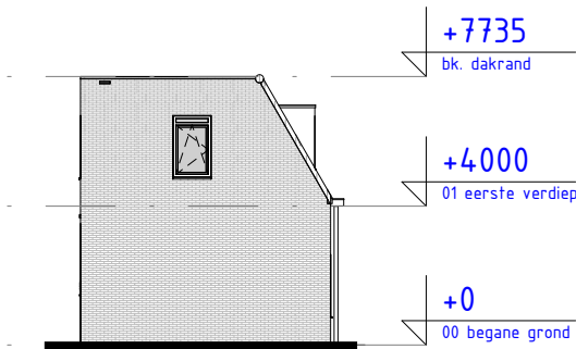
Rechtergevel
