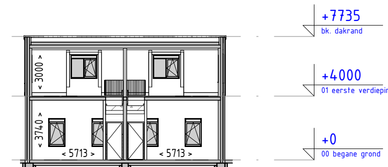
Langsdoorsnede
