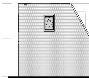
Rechtergevel
