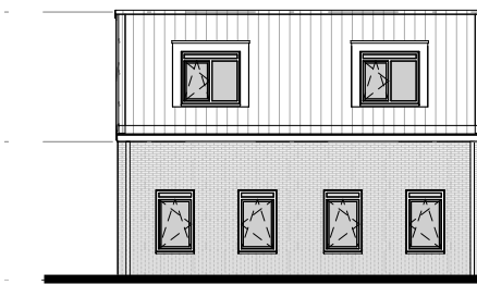
Achtergevel
