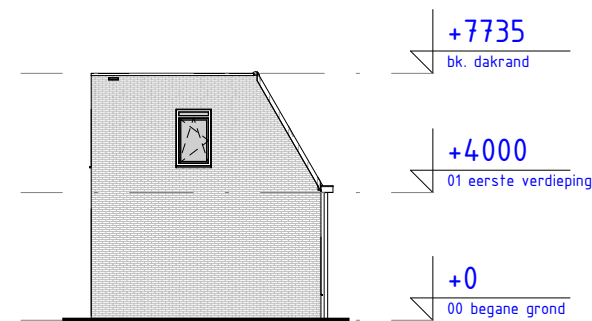
Rechtergevel
