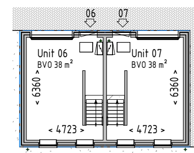
Begane grond
