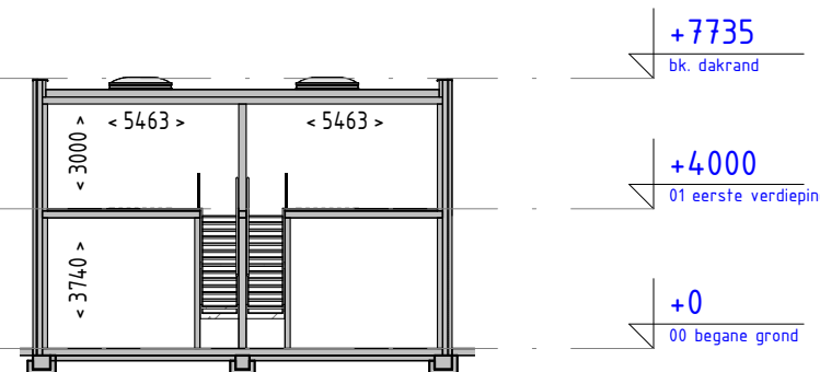
Langsdoorsnede
