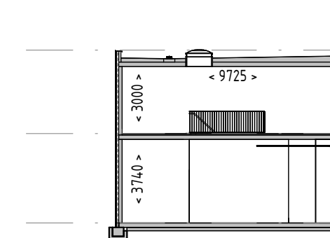
Dwarsdoorsnede
