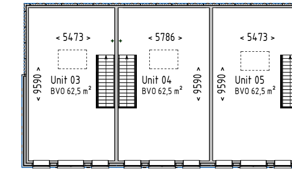
Eerste verdieping
