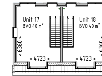
Eerste verdieping
