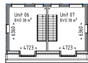
Eerste verdieping
