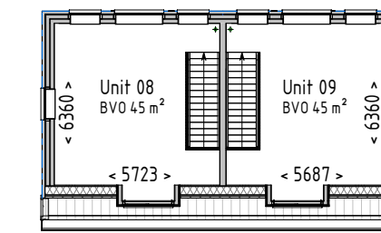
Eerste verdieping
