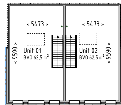
Eerste verdieping
