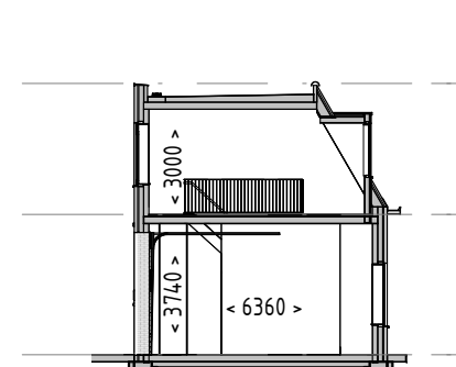
Dwarsdoorsnede
