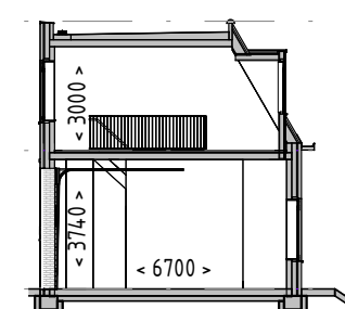
Dwarsdoorsnede
