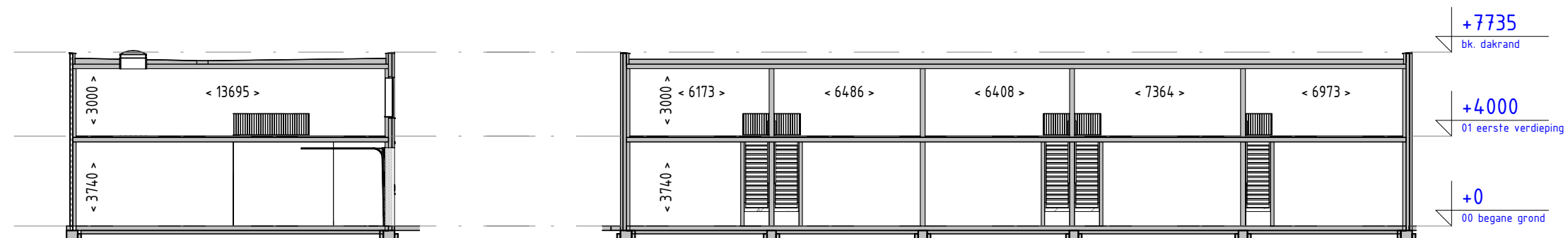
Dwarsdoorsnede
