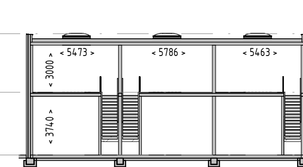
Langsdoorsnede
