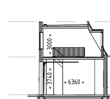
Dwarsdoorsnede
